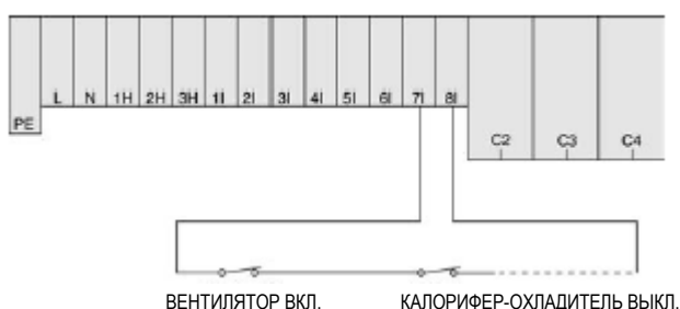
ДИСТАНЦИОННОЕ ВКЛЮЧЕНИЕ/ВЫКЛЮЧЕНИЕ (НОРМАЛЬНО ЗАМКНУТЫЙ КОНТАКТ)
